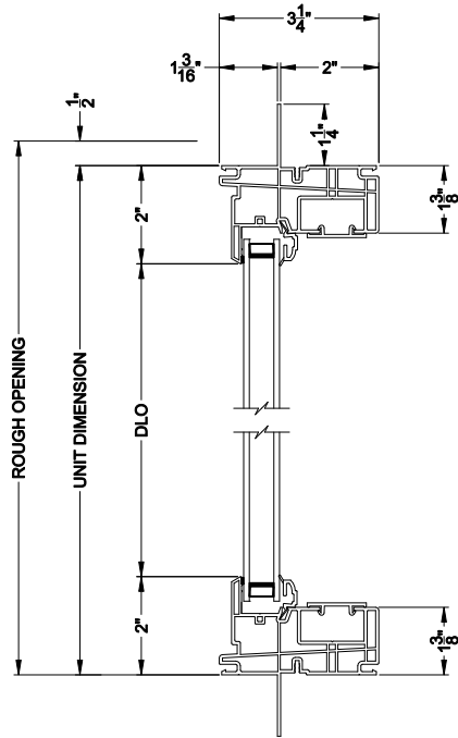
3500 DH PIC / TRANS WINDOW (9310) Vertical Section
