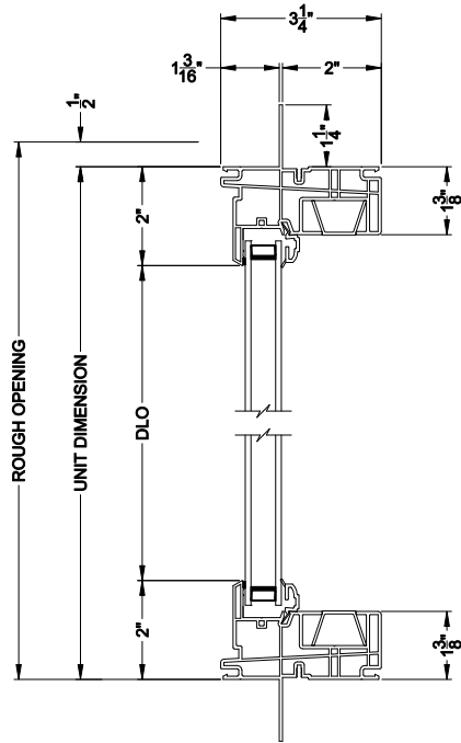
3500 DH PIC / TRANS WINDOW (9310) Vertical Section - Non J-Channel
